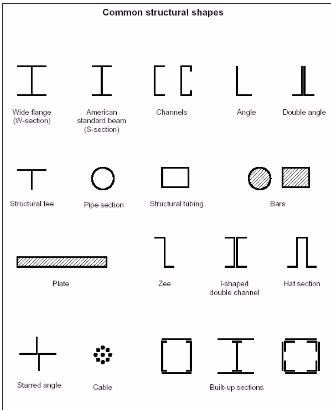
รูปที่ 1.3(ต่อ) แสดงหน้าตัดเหล็กรูปร่างต่างๆ(มาตรฐาน AISC.)
