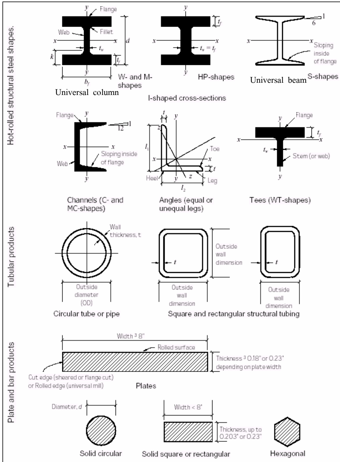
รูปที่ 1.3 แสดงหน้าตัดเหล็กพรรณต่างๆ(มาตรฐาน AISC.)
