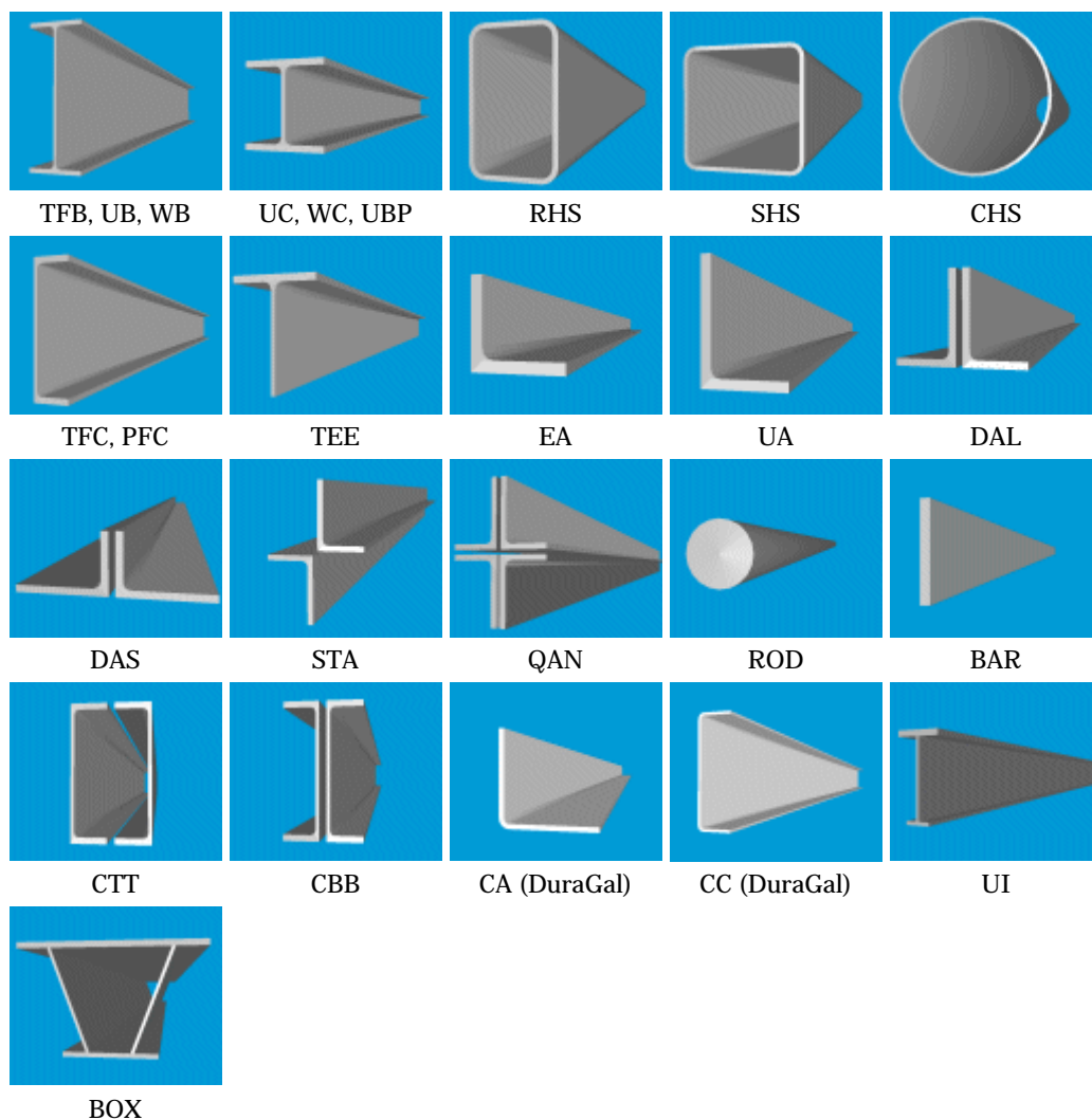
รูปที่ 1.5 แสดงหน้าตัดเหล็กตามมาตรฐานของประเทศต่างๆ
